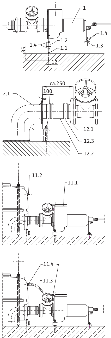
Рис. 4: монтаж насосов
