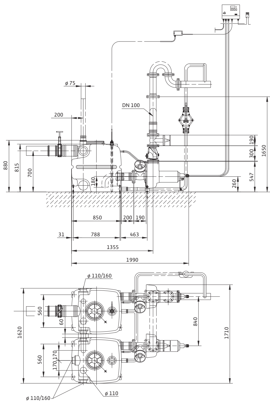
Рис. 2: DrainLift XXL 1080
