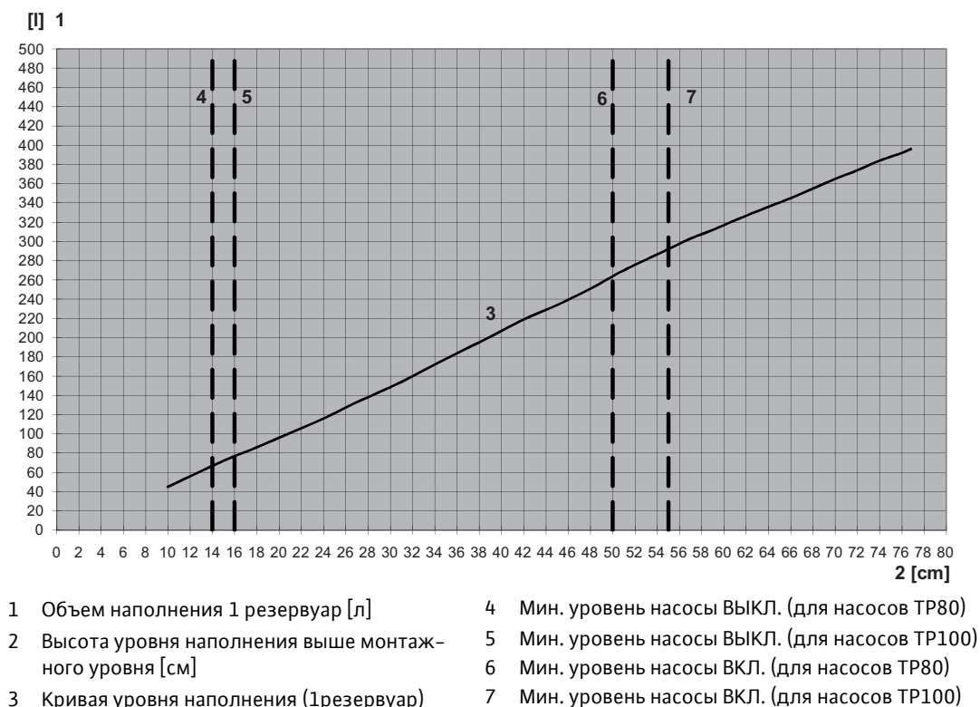
Рис. 10: объем резервуаров в зависимости от уровня наполнения
