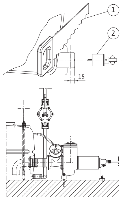
Рис. 8: подключение аварийного спускного отверстия (ручной мембранный насос)
