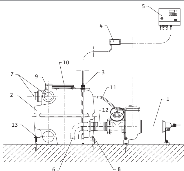
Рис. 1: описание установки
