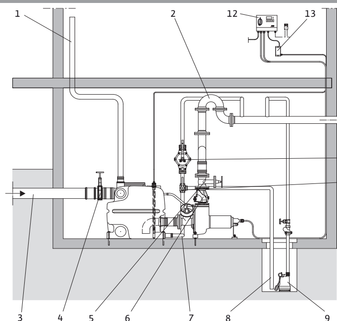
Рис. 9: пример инсталляции
